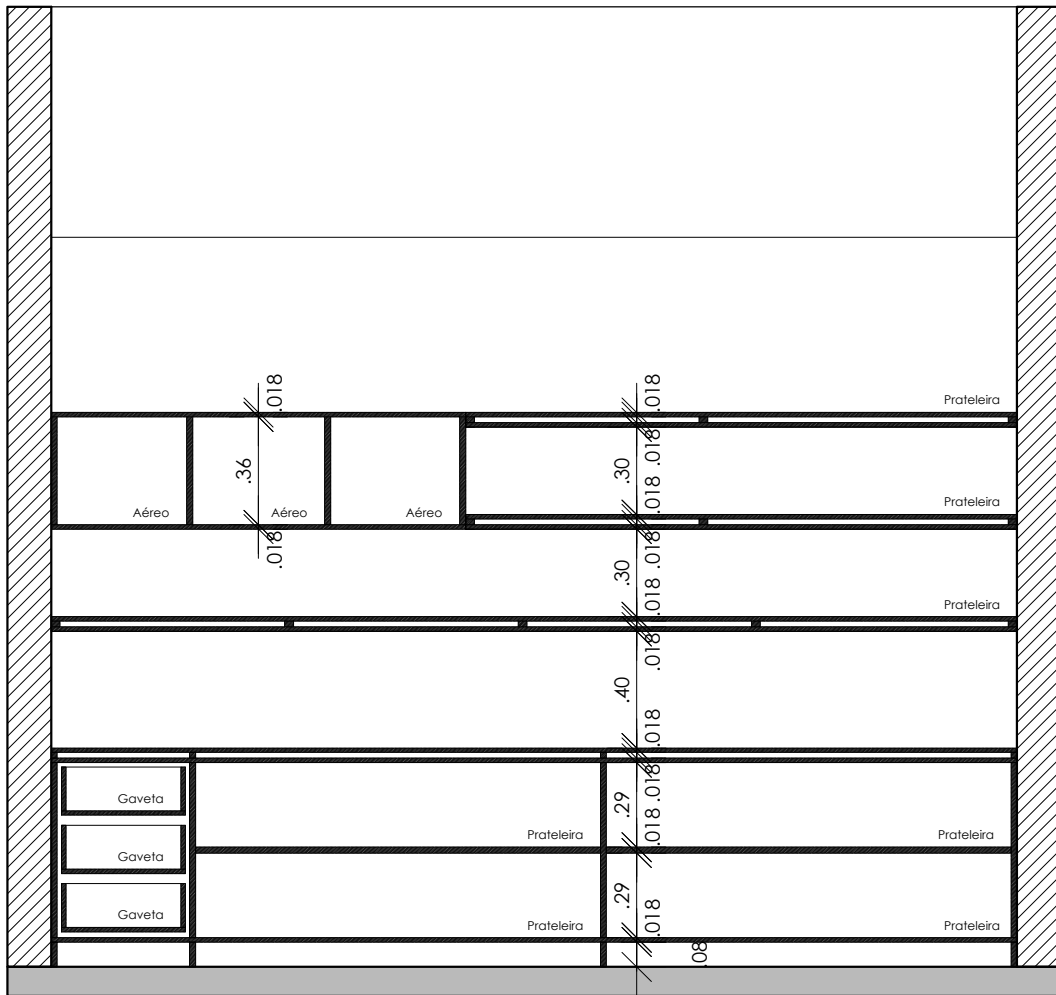
Corte BB Móvel 02 - Sala de Apoio
