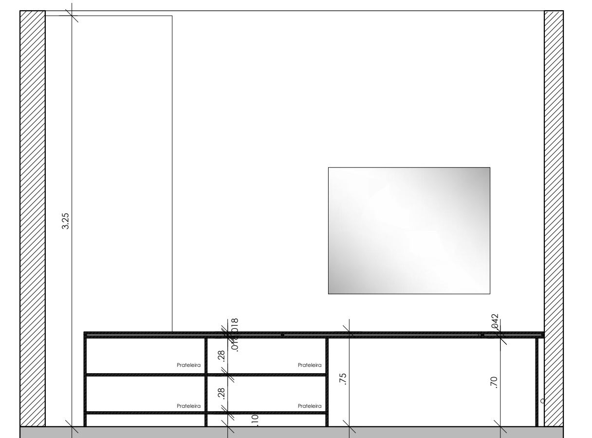
Corte BB Móvel 02- Recepção
