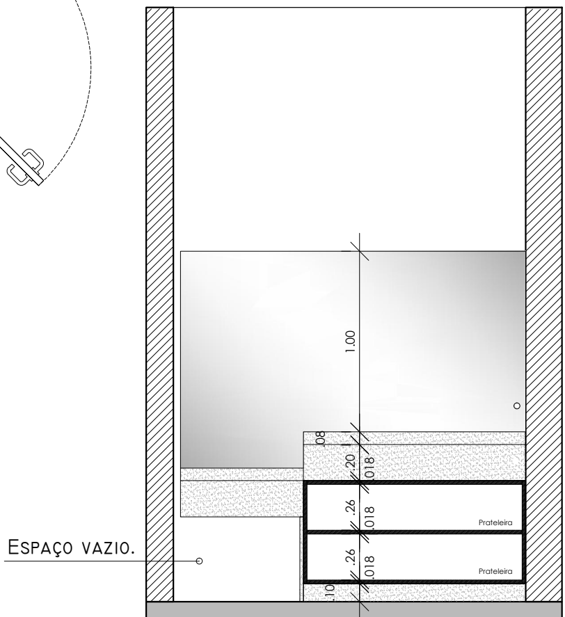
Corte AA WC Masculino
