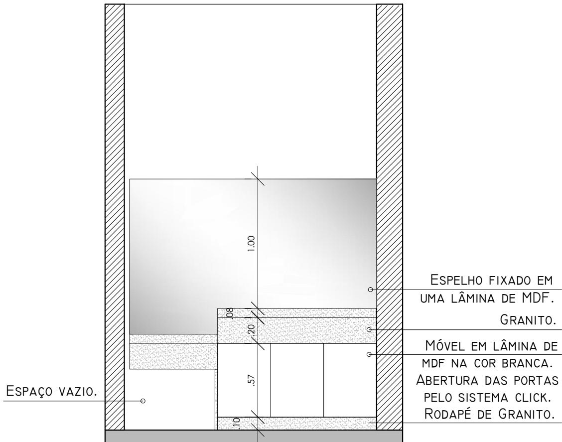
Vista WC Masculino
