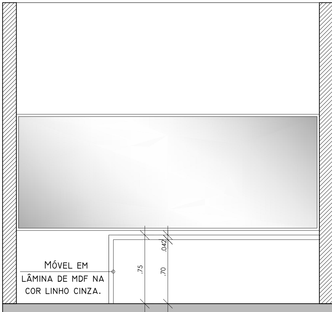
Vista Móvel 01 - Sala de Apoio
