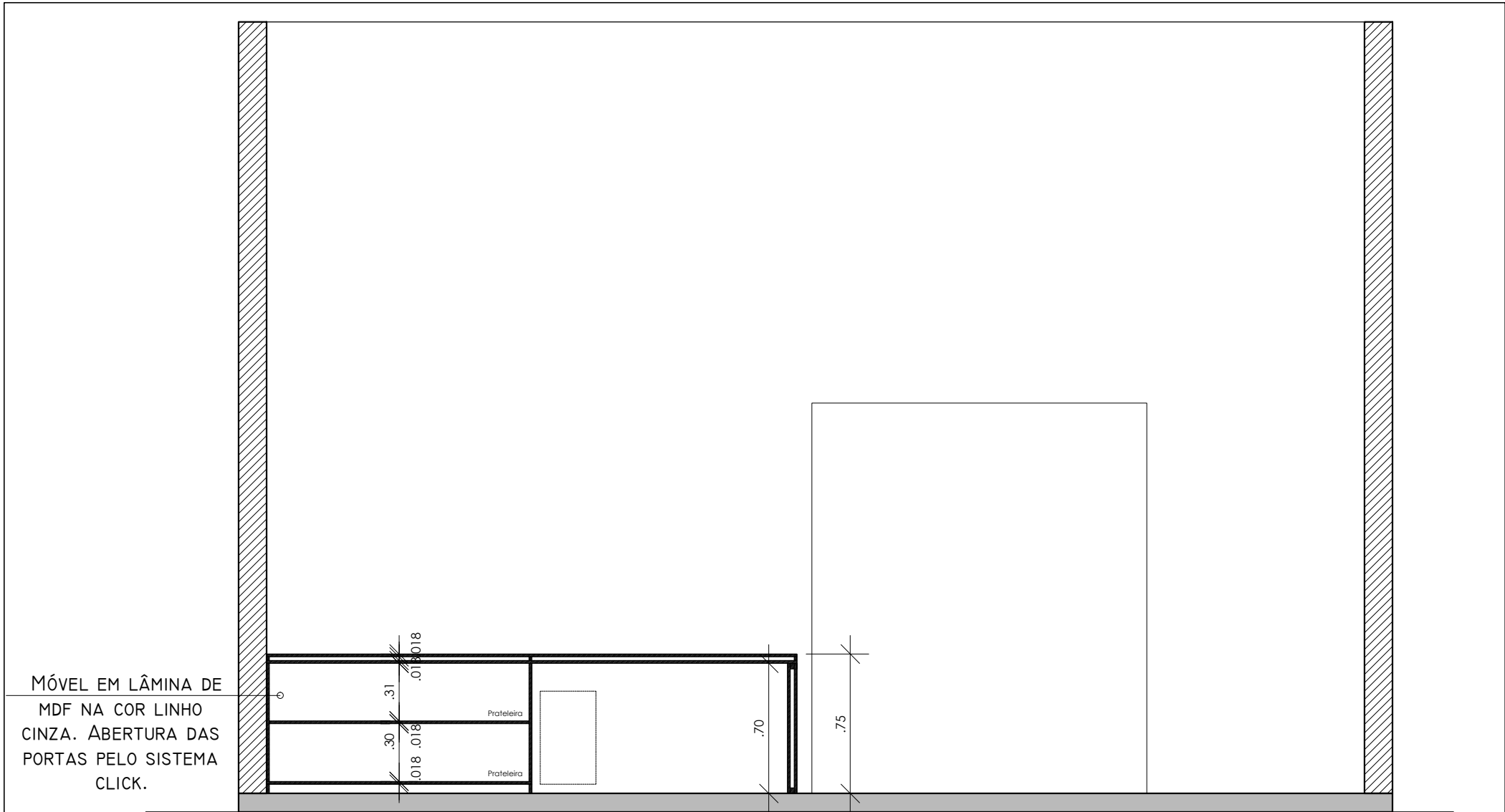
Corte CC Móvel 03- Plenário
