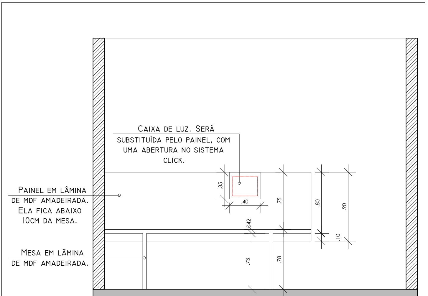
Vista Móvel 01 - cozinha
