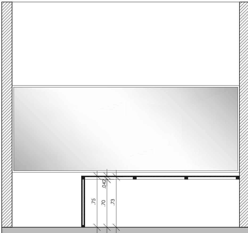
Corte AA Móvel 01 - Sala de Apoio
