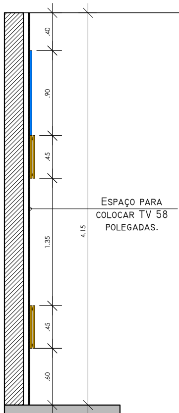
Corte AA Móvel 01 (Painel)- Foyer
