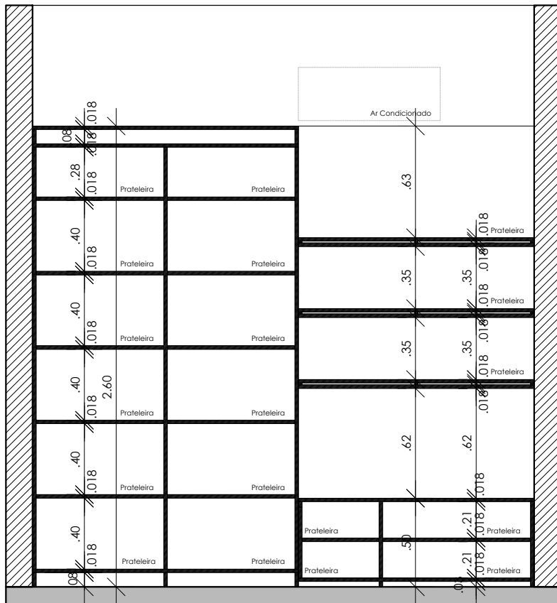
Corte AA Vista 01 - Sala de Assessoria Juridica
