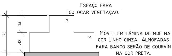
Vista Móvel 02- Foyer
