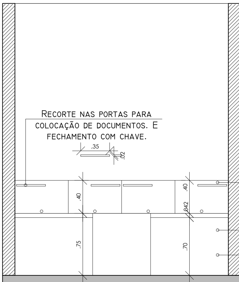
Vista Sala de Vereadores 01 e 02
