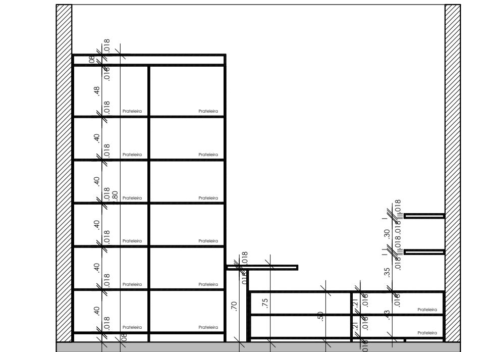
Corte AA Vista 01 - Sala da Tesouraria
