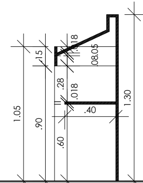
Corte BB Móvel 02 - Plenário
