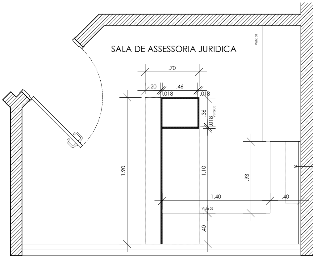
Planta Baixa Sala de Assessoria Juridica - S/Escala
