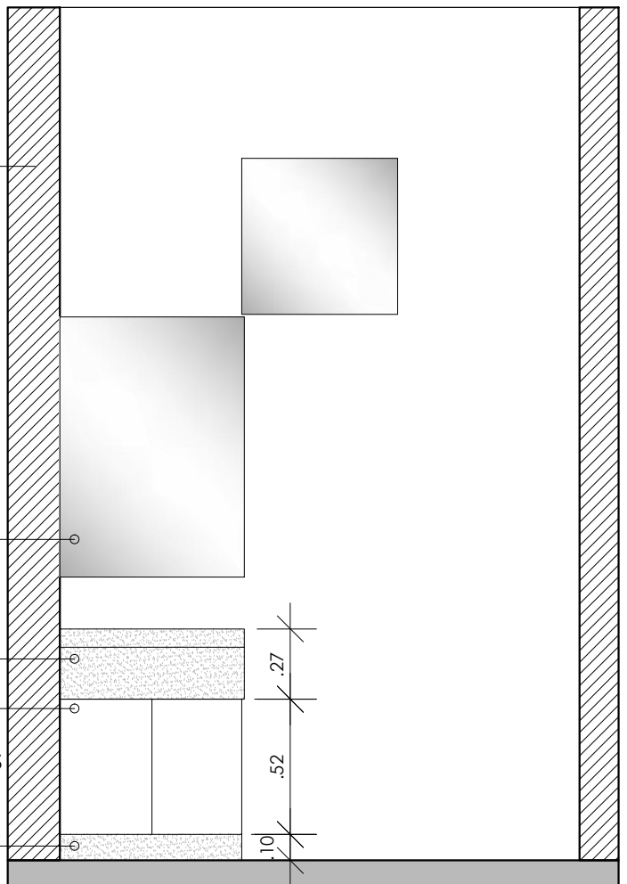
Vista WC Feminino
