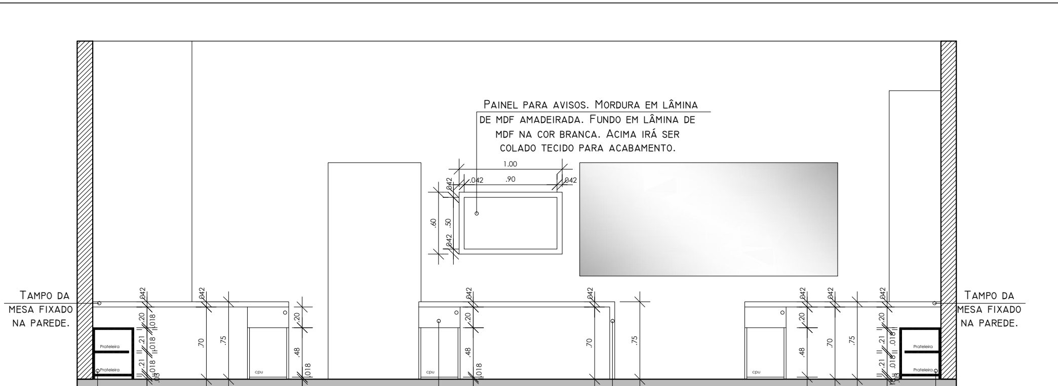
Vista 03 - Sala da Tesouraria
