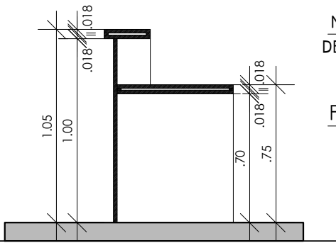
Corte AA Móvel 01 - Recepção
