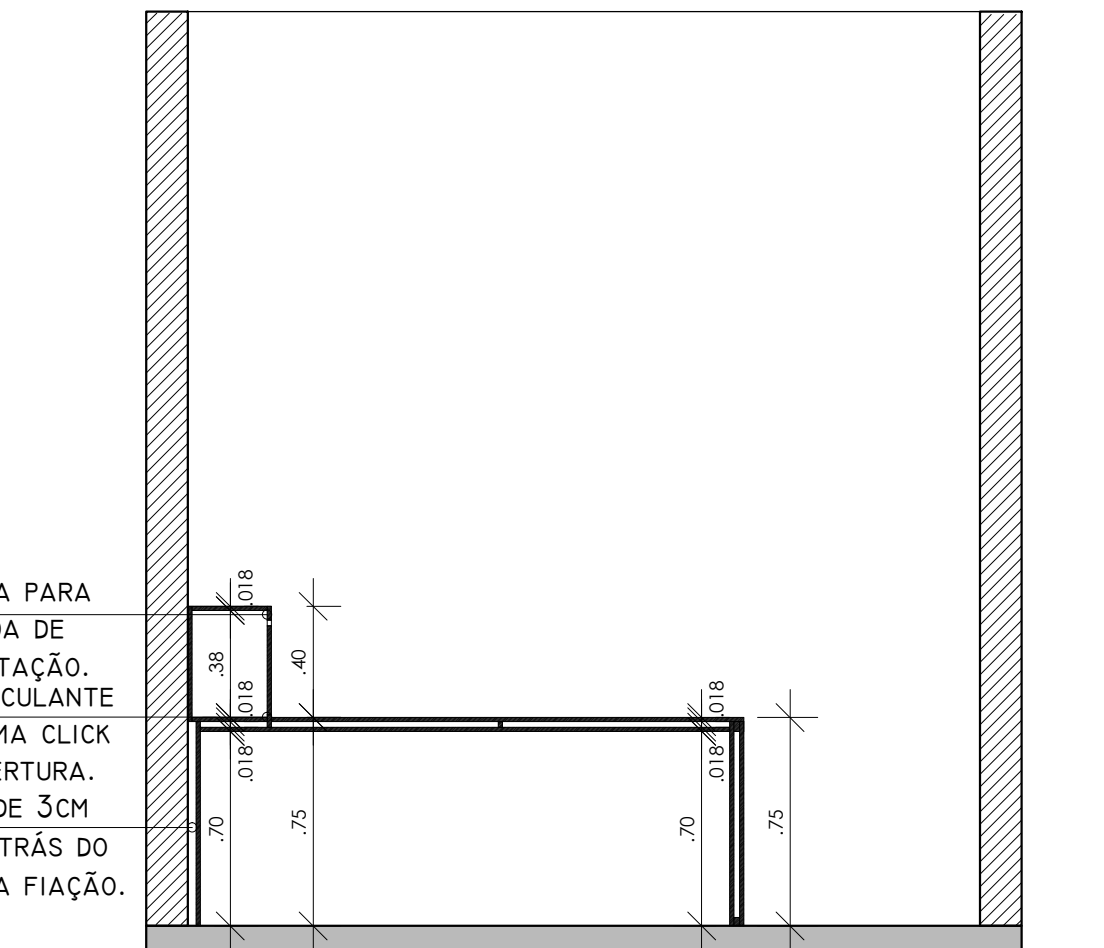
Corte AA Sala de Vereadores 01 e 02
