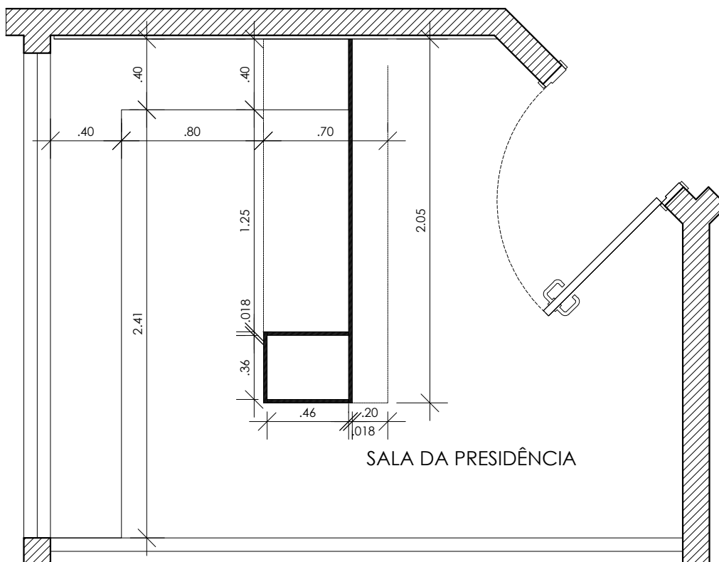
Planta Baixa Sala Presidência - S/Escala
