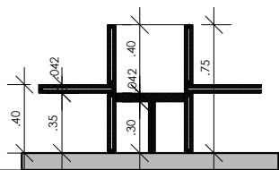
Corte BB Móvel 02- Foyer
