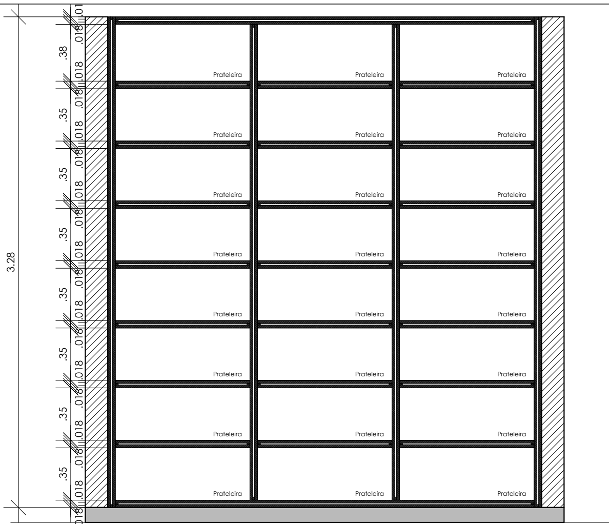
Corte AA Móvel 01- Sala de Arquivo
