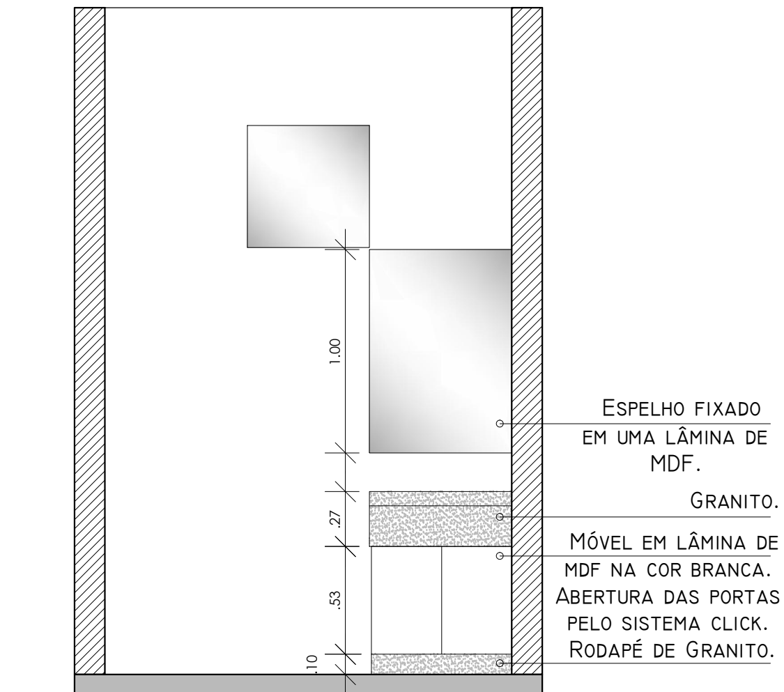
Vista WC Masculino
