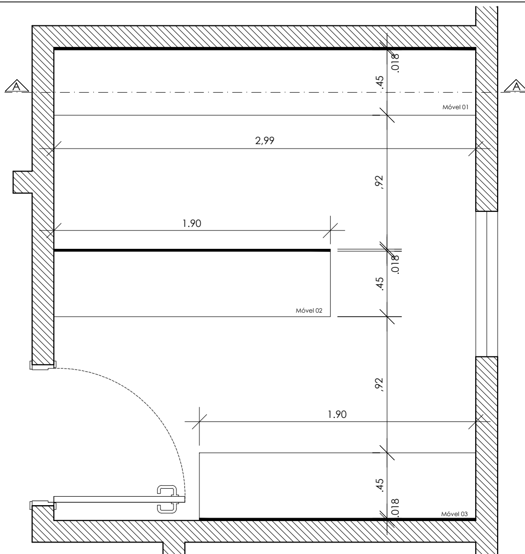
Planta Baixa Sala de Arquivo - S/Escala
