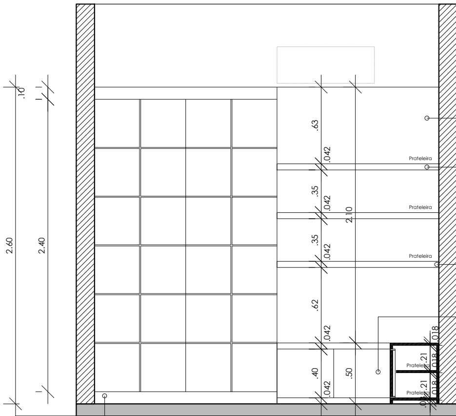
Vista 01 - Sala de Assessoria Juridica
