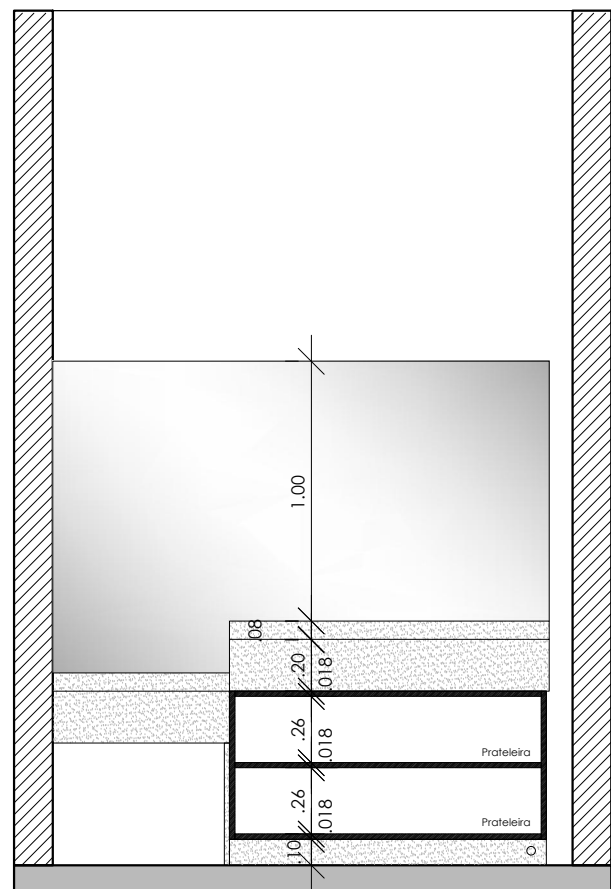
Corte AA WC Feminino
