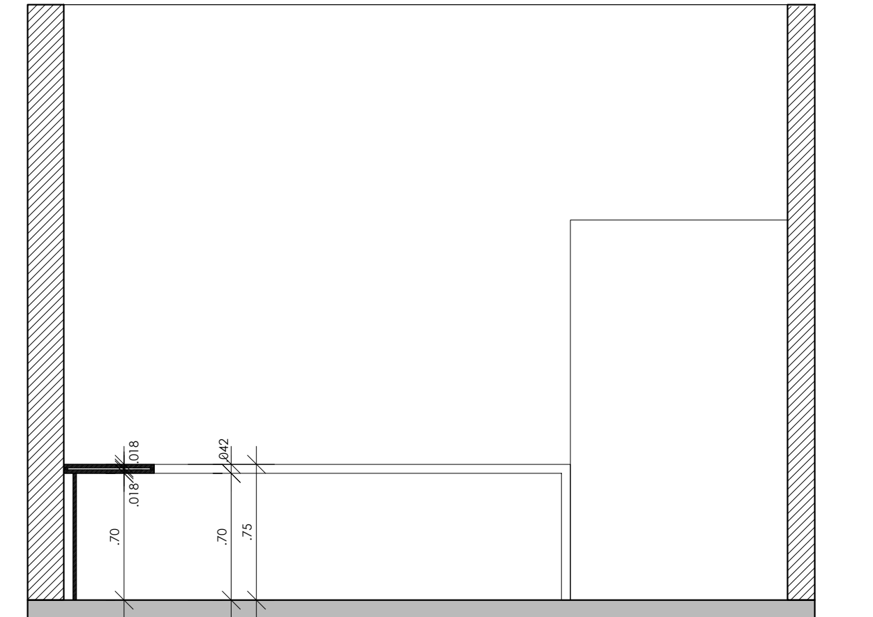
Vista 02 Móvel 02- Recepção
