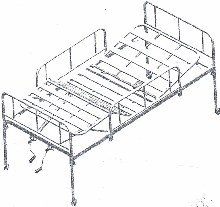
Imagem 5: Linha de cama hospitalar com dois movimentos.
