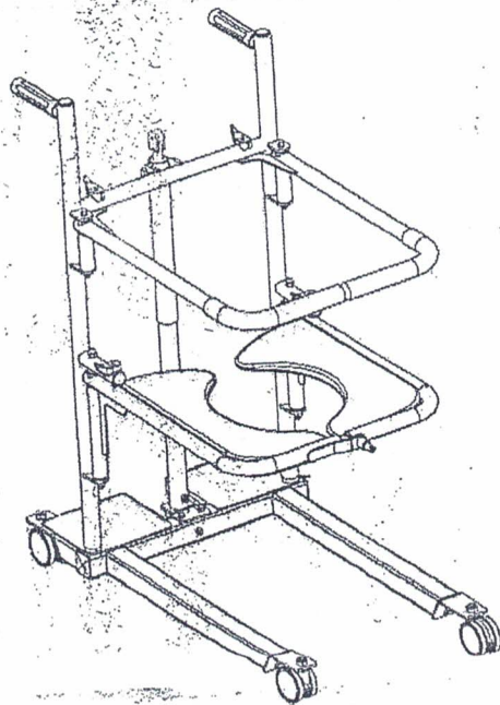
Imagem 7: Linha de Cadeira de Transferência
